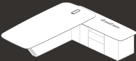
2060×2200×750 2360×2394×750 2660×2452×750
